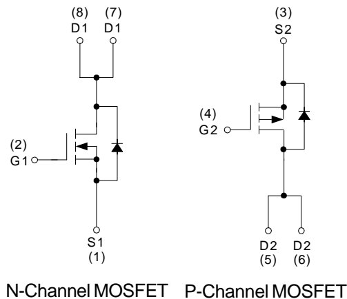
N-Channel MOSFET P-Channel MOSFET
